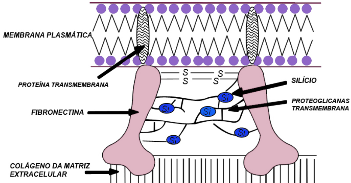
Figura 4. Teor de Silício em humanos.
