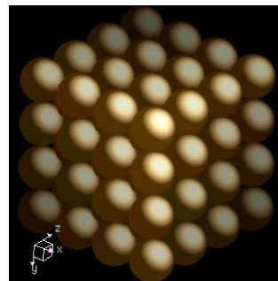
Figura 9. Estrutura do ferro.
