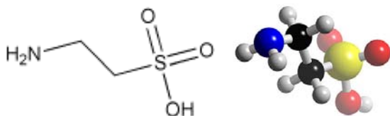
Figura 5. Estrutura química da taurina nas versões plana e 3D.
