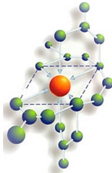
Figura 1. Estrutura dos aminoácidos essenciais.
