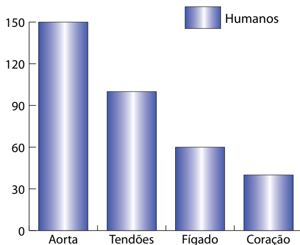
Figura 3. Teor de Silício em humanos.
