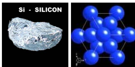
Figura 2. Estrutura do silício.
