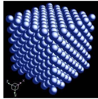
Figura 8. Estrutura do cobre.
