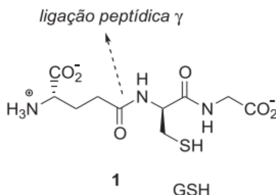
Figura 1: Glutationa (I): \gamma -L-glutamil-L-cisteinilglicina
